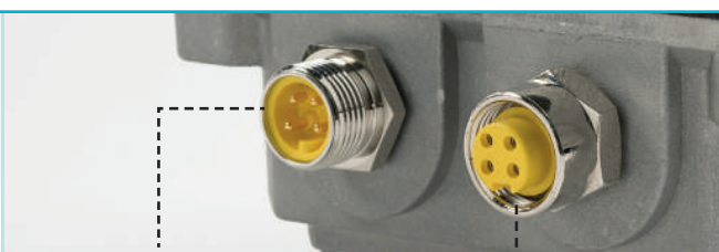
IxI4 Connettore di Alimentazione 3P+E IP67
