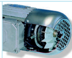
EBDC Autofrenante con freno DC
