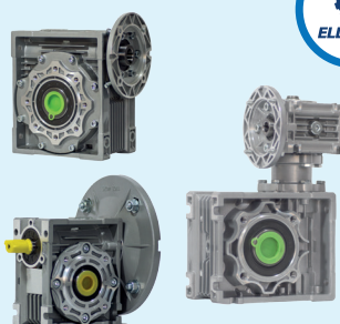
RIDUTTORI A VITE SENZA FINE (MRDV)
