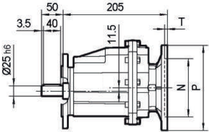
II Ø160
