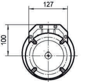
III Ø200
