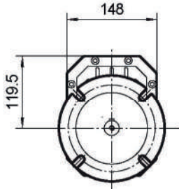
III Ø250
