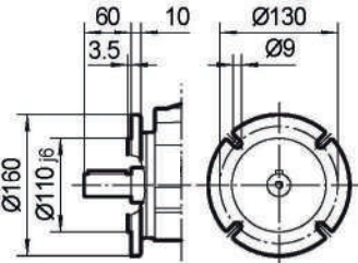
I Ø160
